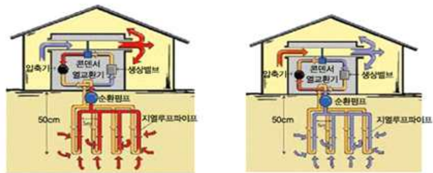
<< 지열에너지 개념도 >>
