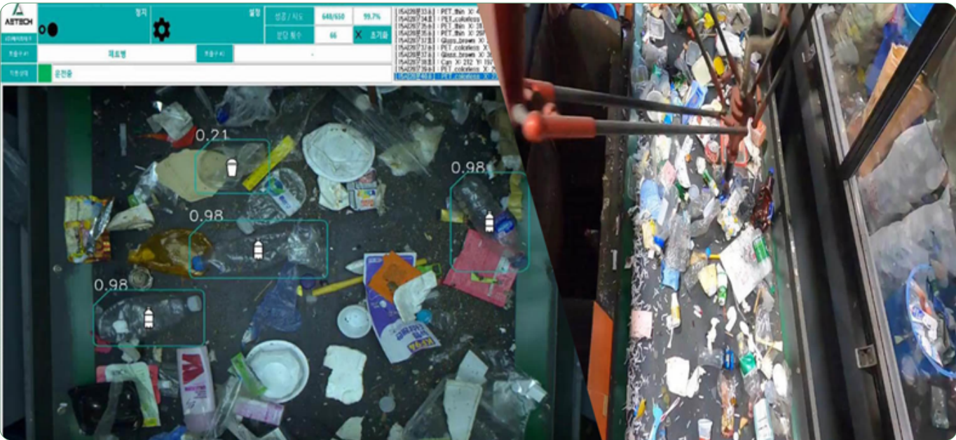
▲ AI 폐기물 선별 로봇이 컨베이어 벨트에서 폐기물 종류를 구별한 후, 재활용이 가능한 페트병을 흡착하여 옮기고 있다. 출처 : 에이트테크
